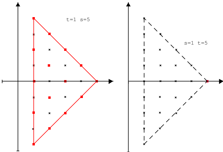
FIGURE 1. Les points marqués d'un carré donnent les coordonnées (r, i) des m_{s,t}(r, i) = 1 dans le cas d'une Speh ( t = 1 ) à gauche et d'une Steinberg ( s = 1 ) à droite
