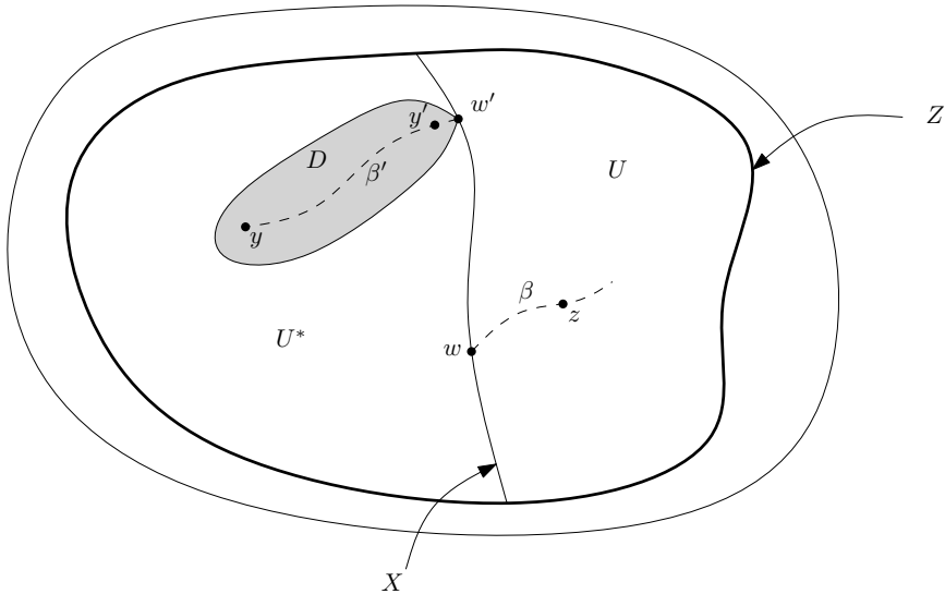
FIGURE 2.1. Démonstration de la proposition 2.12'
