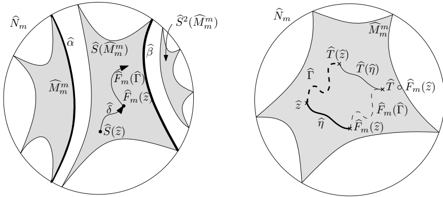
FIGURE 3.1. Démonstration du lemme 3.4
