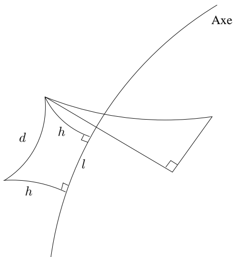
FIG. 2.2. Illustration du lemme 2.2
