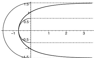
FIG. 2.1. Les ouverts \mathcal{B}_{\ln(2)} \subset \Delta \subset \mathcal{B}_{\frac{\pi}{2}} .
